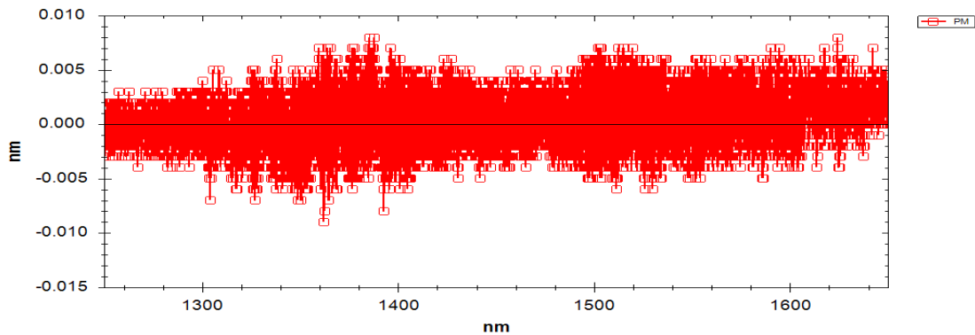
1250-1650波长准确性
