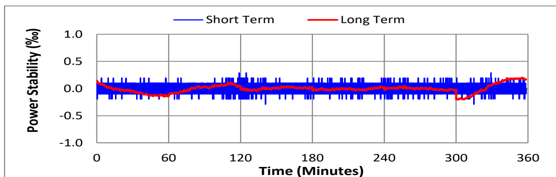
6小时功率稳定性
